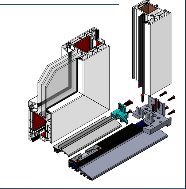
Capac prag PM - profil MD
